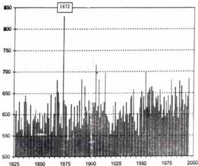
Entwicklung der jährlichen Höchstwasserstände am Pegel Travemünde seit 1825
